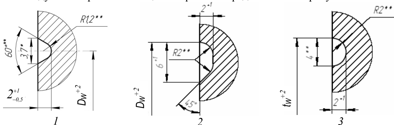
1 – проточка по диаметру; 2 – проточка по диаметру; 3 – проточка по толщине обода
